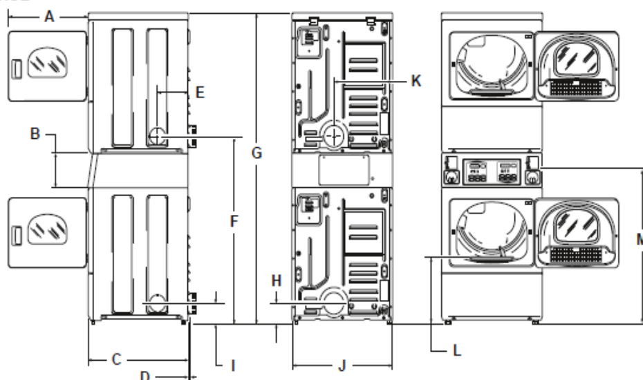
модель NSE
